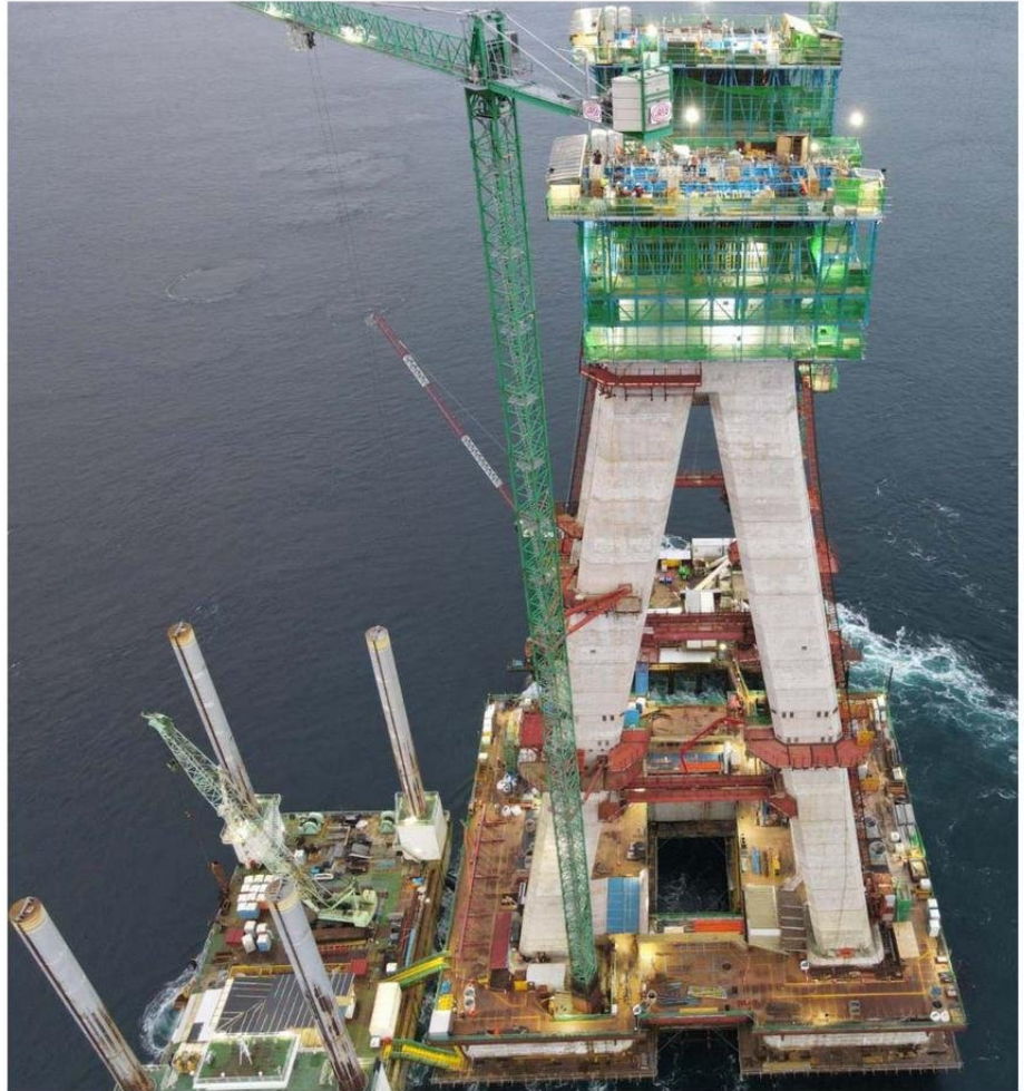
LA CONSTRUCCIÓN DE LOS PILARES DEL PUENTE CHACAO REGISTRAN UN IMPORTANTE AVANCE DESTACADO POR LA COMUNIDAD Y AUTORIDADES.
