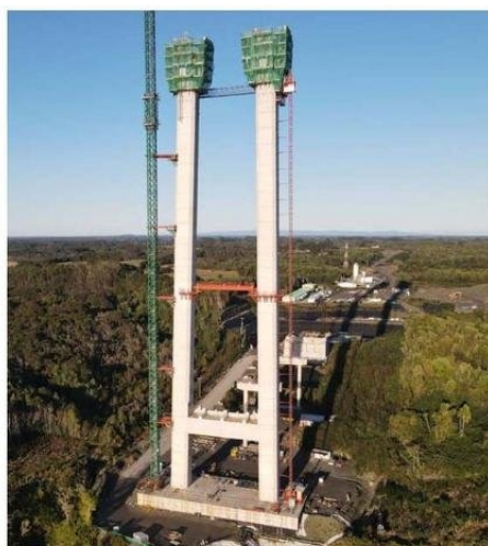
PILA SUR: LA ESTRUCTURA QUE ESTÁ EN TIERRA LLEVA 152,7 METROS.
