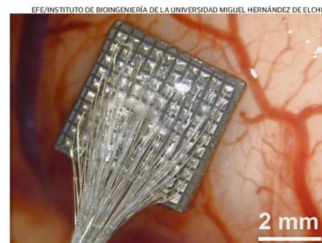
MATRIZ DE 100 MICROELECTRODOS EN CORTEZA CEREBRAL HUMANA.
