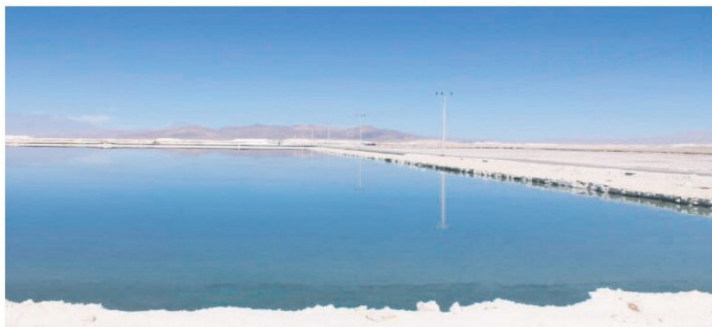
Piscinas de evaporación de litio de la empresa SQM en el Salar de Atacama. / CORTESÍA BARINIA MONTVOYA
