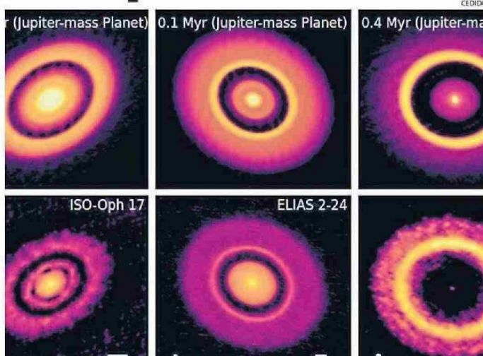
AL COMBINAR OBSERVACIONES Y SIMULACIONES, SE PUDO RASTREAR CÓMO LOS PLANETAS PUEDEN FORMARSE Y REMODELAR SUS DISCOS.
