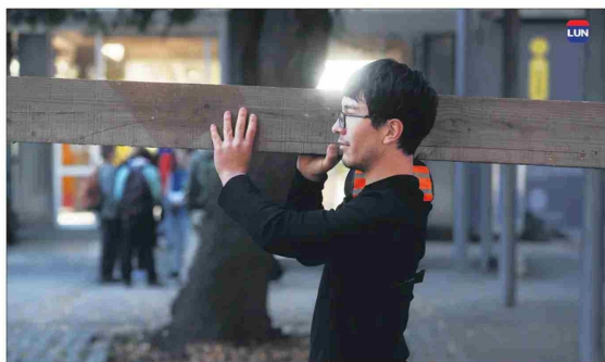
La hombrera con celdas de carga incorporadas que detectan el exceso de peso.
