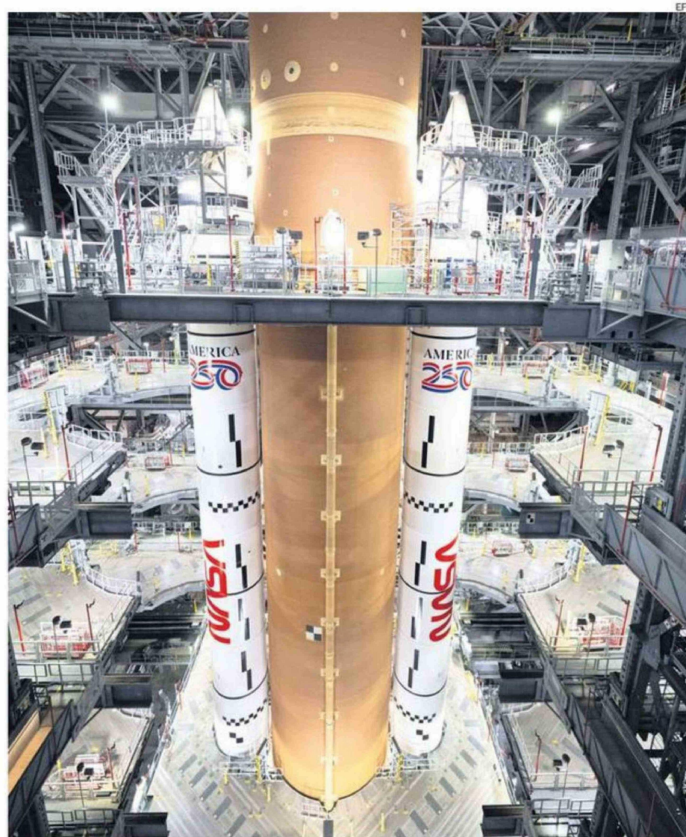
COHETE DEL SISTEMA DE LANZAMIENTO ESPACIAL (SLS) DE LA MISIÓN ARTEMIS II EN EL CENTRO ESPACIAL KENNEDY.
