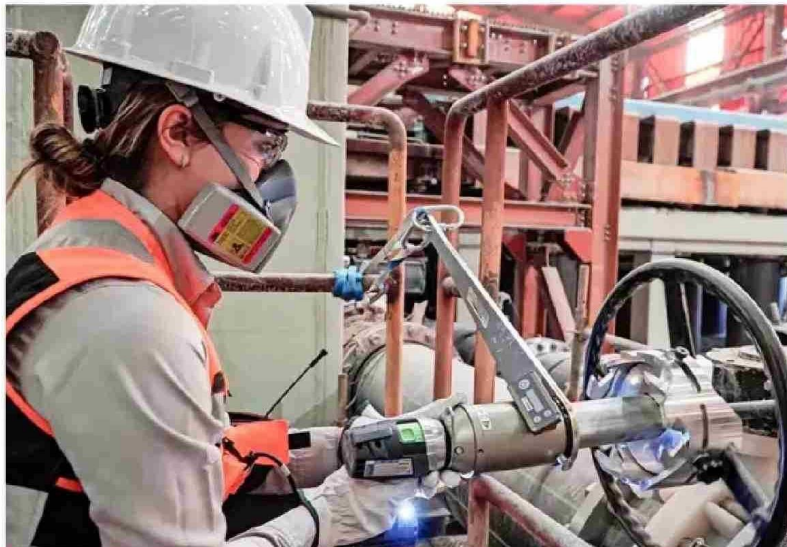
La División Gabriela Mistral de Codelco instaló un actuador portátil mecánico, que reemplaza tareas que demandaban un alto esfuerzo.
