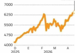
Kospi
