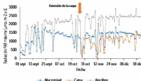
Figura 6. Radiación fotosintéticamente activa (PAR) máxima bajo macrotúnel, carpa y aire libre en Molina, región del Maule, 2025.
