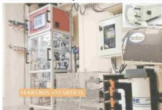
Sistema FerryBox de monitoreo oceanográfico autónomo.
