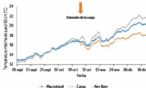
Figura 5. Temperatura mínima de suelo a los 60 cm de profundidad bajo macrotúnel, carpa y aire libre en Molina, región del Maule, 2023.
