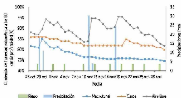
Figura 7. Evolución de la humedad en el suelo en macrotúnel, carpa y al aire libre, y lámina de riego aplicada en cv. Santina, región del Maule, 2025.
