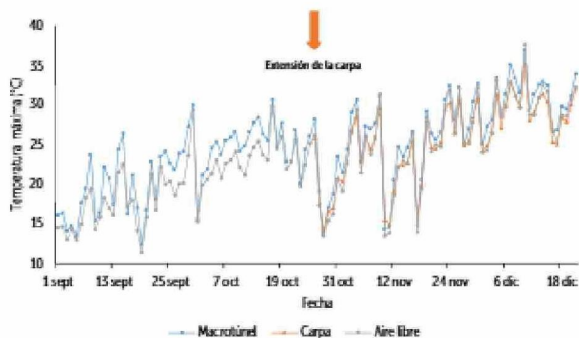
Figura 2. Temperatura máxima de suelo a los 40 cm de profundidad bajo macro túnel, carpa y aire libre en Molina, Región del Maule, 2023.
