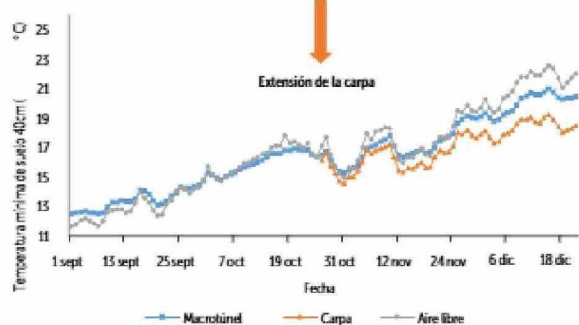
Figura 3. Temperatura mínima de suelo a los 40 cm de profundidad bajo macro túnel, carpa y aire libre en Molina, región del Maule, 2023.
