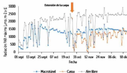
Figura 6. Radiación fotosintéticamente activa (PAR) máxima bajo macrotúnel, carpa y aire libre en Molina, región del Maule, 2023.
