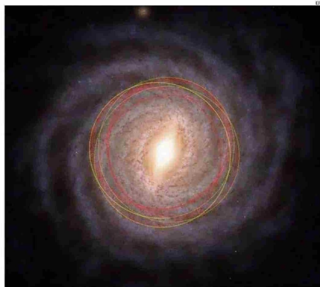
3I/ATLAS ES EL TERCER OBJETO CONOCIDO PROCEDENTE DE FUERA DEL SISTEMA SOLAR QUE SE HA SIDO AVISTADO.
