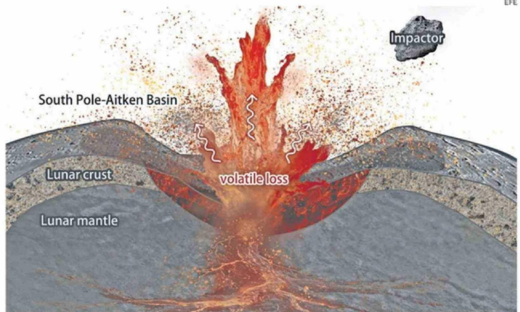
ILUSTRACIÓN DEL IMPACTO DE UN METEORITO QUE FORMÓ LA CUENCA AITKEN EN LA CARA OCULTA DE LA LUNA.
