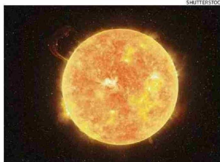
UNA IMAGEN DEL SOL CAPTADA POR LA NASA.
