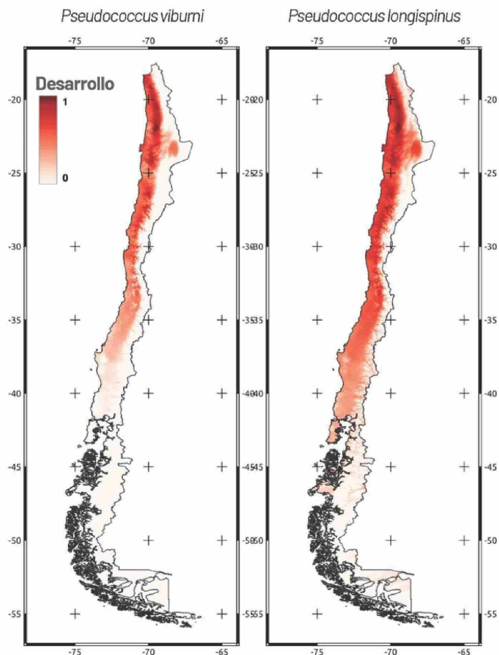
Proyección de la distribución de dos especies de chanchito blanco bajo escenarios de cambio climático.
