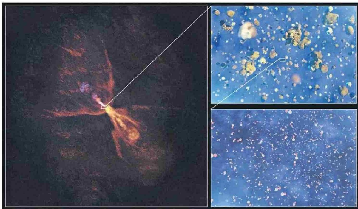
Formación de silicatos alrededor de la estrella bebé HOPS-315.
