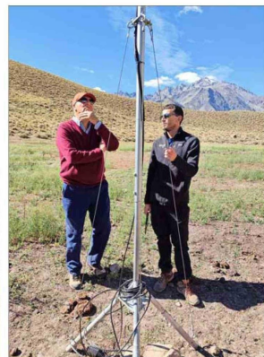
Para el monitoreo de aguas subterráneas se instalaron antenas de transmisión satelital como esta.
