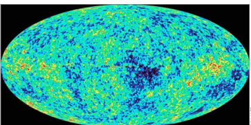
"Descubrimientos como el Big Bang permiten un diálogo fecundo entre disciplinas con distintos objetivos, como la cosmología, la filosofía y la teología". Imagen de la Nasa con las zonas antiguas y nuevas del Universo.
