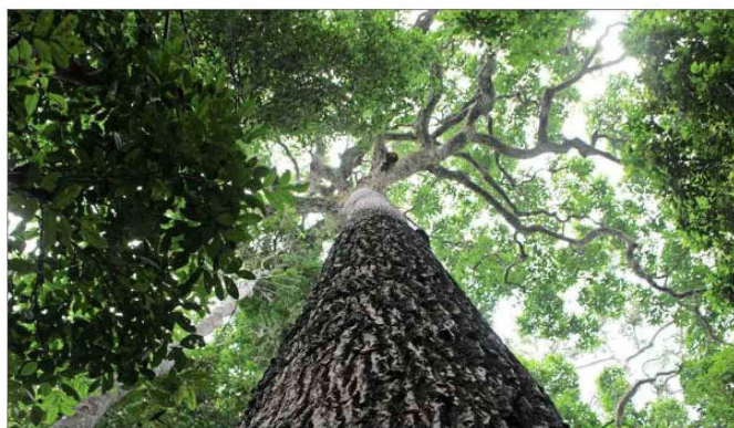
La Amazonia experimentó su mayor pérdida de cubierta arborea desde 2016, dice el informe del Global Forest Watch.
