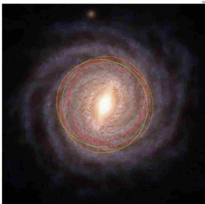
3I/ATLAS ES EL TERCER OBJETO CONOCIDO PROCEDENTE DE FUERA DEL SISTEMA SOLAR QUE SE HA SIDO AVISTADO.
