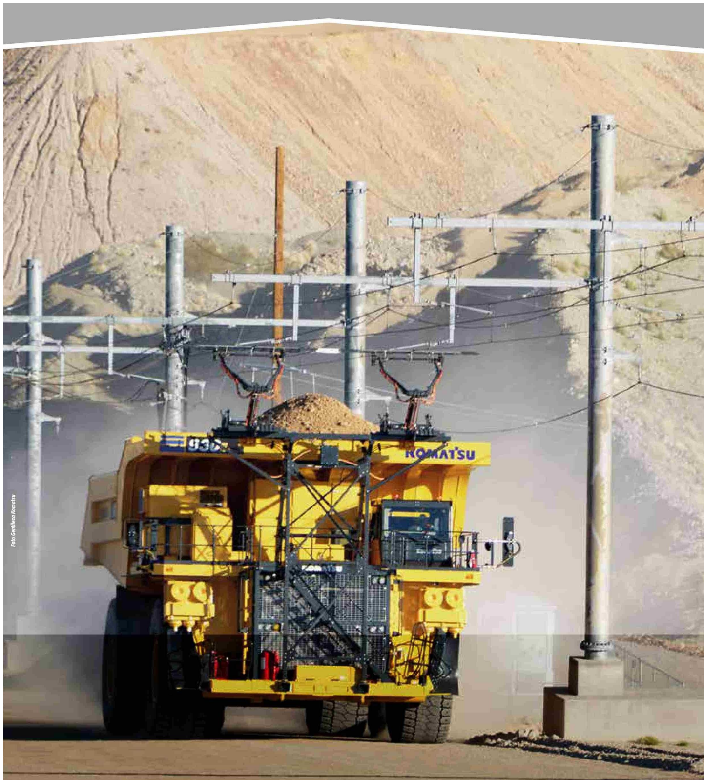
Camión minero Komatsu 930 PADT en operación.
