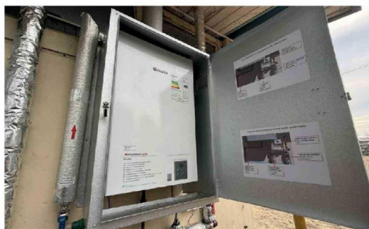
SISTEMA CONSIDERA DOS EQUIPOS TERMOFÓN de 150 litros cada uno, con respaldo mediante calefones y red de distribución interna certificada para abastecer al establecimiento.
