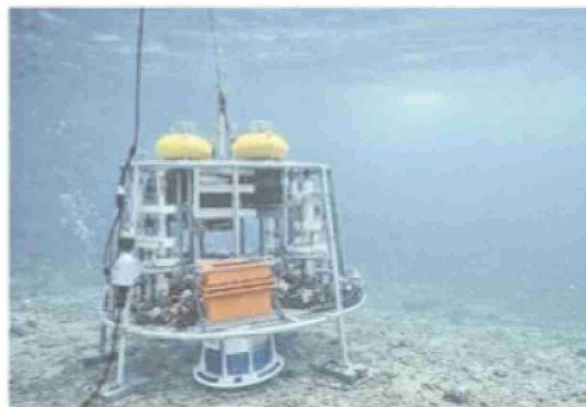
Plataforma submarina multiparamétrica conocida como Lander.
