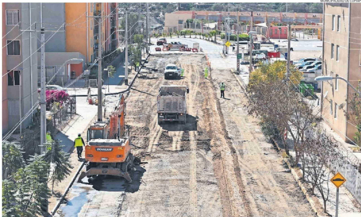
TRABAJOS DE PAVIMENTACIÓN EN AVENIDA LUIS FLORES DURANTE EL 2024 Y QUE ERA PARTE DEL PROYECTO "CONSERVACIÓN DE CALLES Y VÍAS COPIAPÓ III ETAPA".
