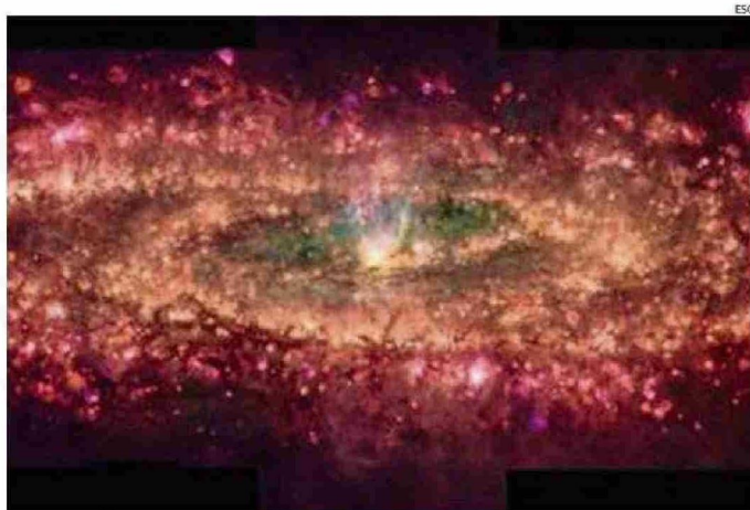
"NGC 253" ESTÁ UBICADA A 11 MILLONES DE AÑOS LUZ DE DISTANCIA.
