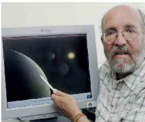
Imagen de archivo del 51 Peg b, que en 1995 descubrieron los astrónomos Michel Mayor (en la imagen) y Didier Queloz, que les valió el Premio Nobel de Física en 2019 y que marcó el inicio de la revolución de los exoplanetas. EFE/EPA/SALVATORE DI NOLFI
