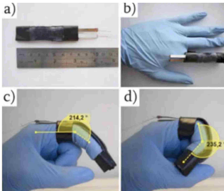
Prototipo del sensor adherido al dedo índice. El dispositivo permite medir la flexión del dedo con gran precisión, detectando variaciones en la capacitancia según el movimiento.
