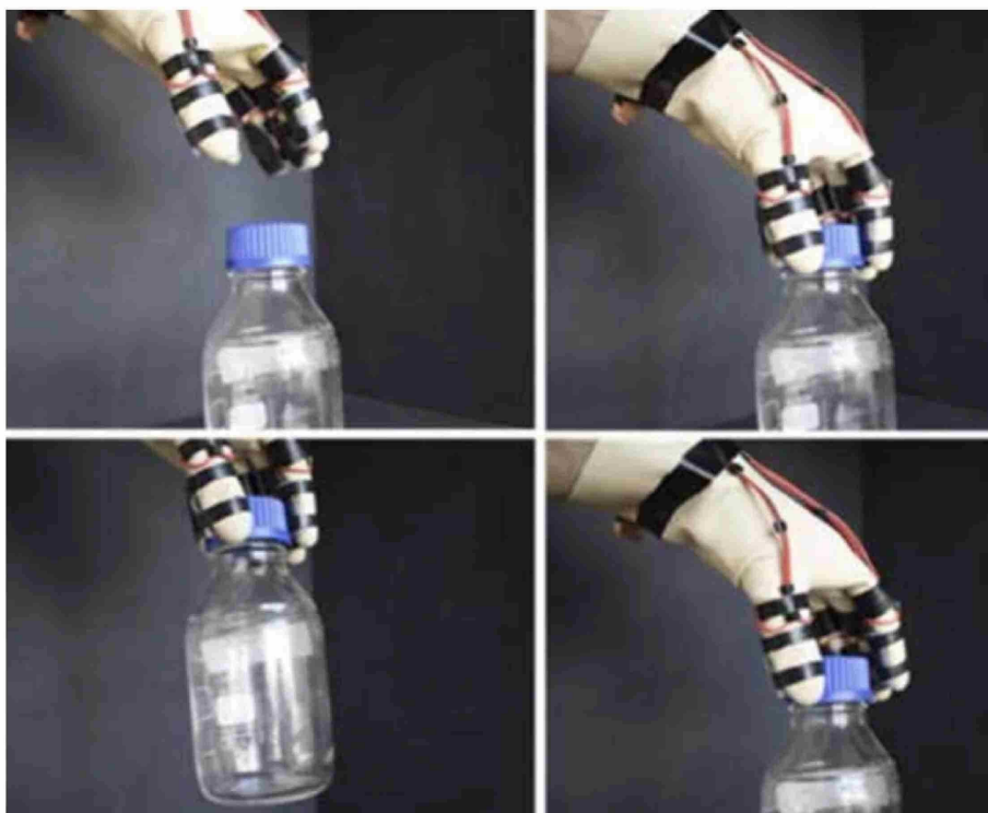
Secuencia del guante inteligente levantando y soltando una botella de vidrio. El sensor detecta el peso aplicado al objeto y transmite los datos en tiempo real, abriendo aplicaciones en robótica, salud y más.
