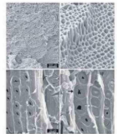
ANATOMÍA DE MADERA FÓSILES CON EVIDENCIA DE INCENDIOS.
