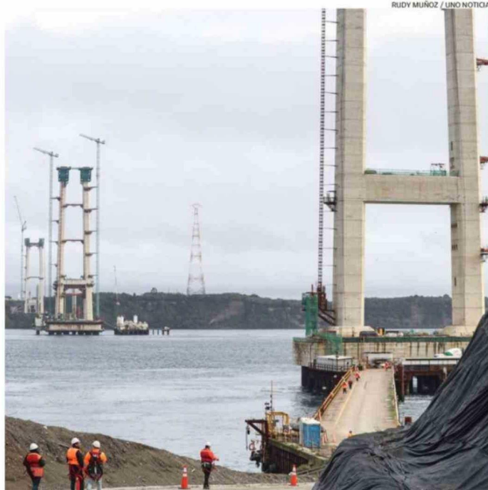
CONTEMPLA LA CONSTRUCCIÓN DE UNA PASARELA A 200 METROS SOBRE EL MAR PARA INSTALAR EL CABLEADO.
