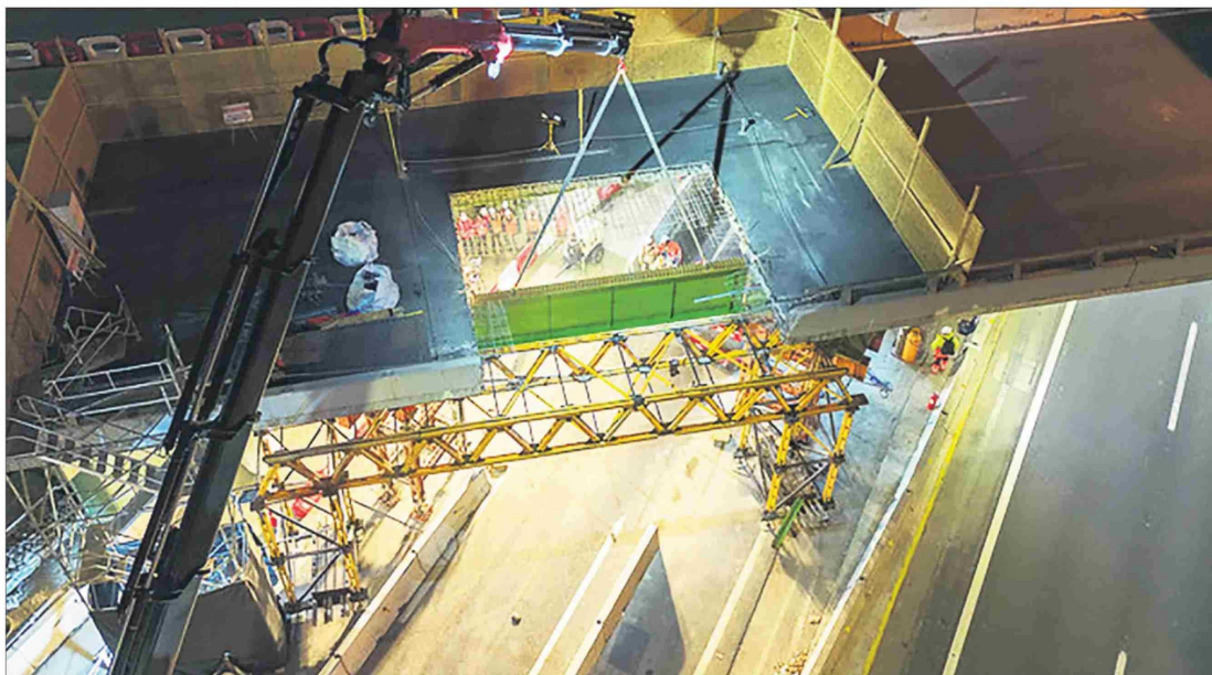
Vista superior del momento en que la grúa instaló el tramo de viga de 7 metros y 3 toneladas la madrugada de este viernes.
