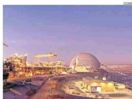
PLANTA DE MINERA SPENCE DE BHP EN LA COMUNA DE SIERRA GORDA.
