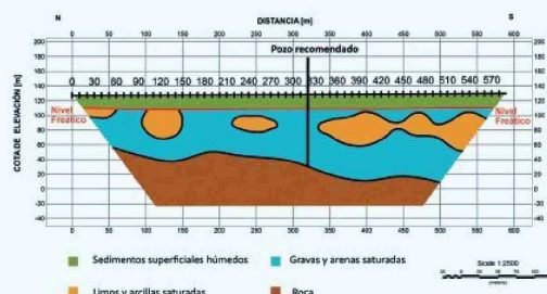
FIGURA 3 Recomendación para la construcción de pozos
