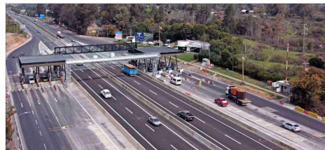
La segunda concesión de Talca-Chillán tiene una longitud de 193 kilómetros y considera diversas obras y mejoras, entre ellas, terceras pistas, pasarelas, 19 puentes y el bajiá Talca.
