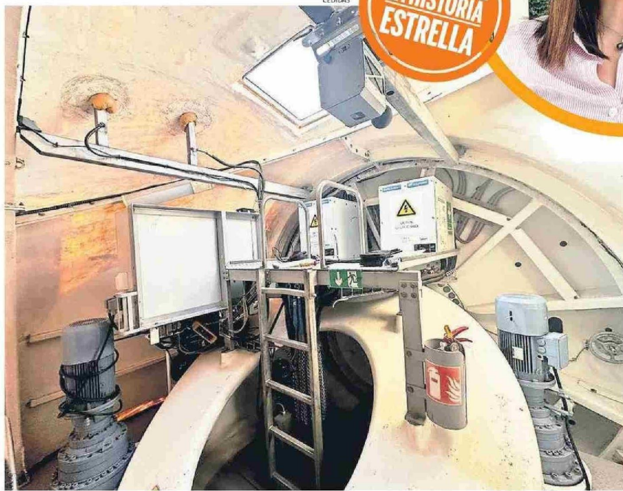
EL SISTEMA ESTÁ INSTALADO DENTRO DE LAS NACELLES (GÓNDOLAS O CABINA) QUE VAN DETRÁS DE LAS HÉLICES DE LAS TORRES EÓLICAS.
