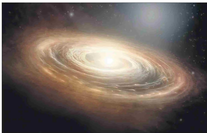
Esta imagen es una representación de un "disco protoplanetario", donde nacen los planetas.
