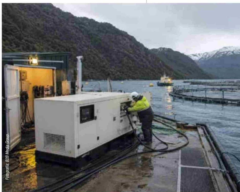
Generadores en operación en salmonicultura.
