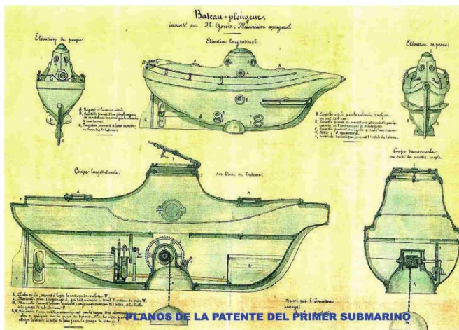
Plano y detalles del malogrado submarino Flach, hundido en la bahía de Valparaíso el 3 de mayo de 1866.
