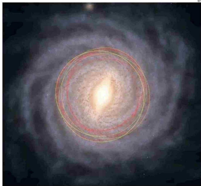
31/ATLAS ES EL TERCER OBJETO CONOCIDO PROCEDENTE DE FUERA DEL SISTEMA SOLAR QUE SE HA SIDO AVISTADO.
