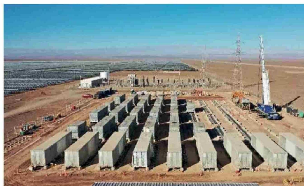
Proyecto BESS de Transelec para Granja Solar de Copec, uno de los sistemas de almacenamiento energético de mayor escala del país, con 420 MWh de capacidad.
