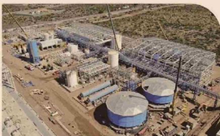
PLANTAS DESALINIZADORAS Foto: IDE Technologies, Aguas Pacífico
