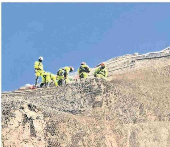
SE HAN INSTALADO 60.086 METROS CUADRADOS DE MALLA METÁLICA PARA EVITAR DERUMBES.
