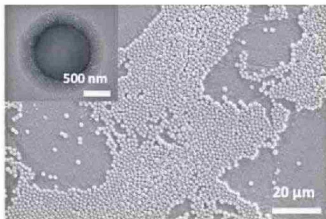
IZQUIERDA: INTERIOR DE CÉLULAS SINTÉTICAS OCUPADAS CON MOLÉCULAS ACTIVAS, QUE HACEN QUE EL SISTEMA EVOLUCIONE QUÍMICA Y FÍSICAMENTE.
