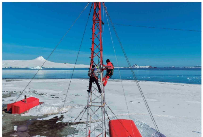
WOM instaló la antena más austral en uno de los lugares más extremos del mundo, el Territorio Chileno Antártico.
