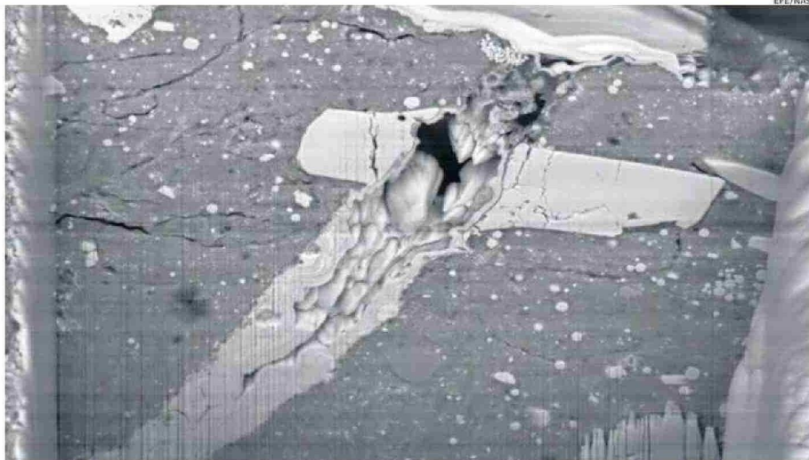
IMAGEN DE MICROSCOPIO ELECTRÓNICO DE BARRIDO DEL CRÁTER DE IMPACTO DE MICROMETEORITO EN UNA PARTÍCULA DE MATERIAL DE BENNU.
