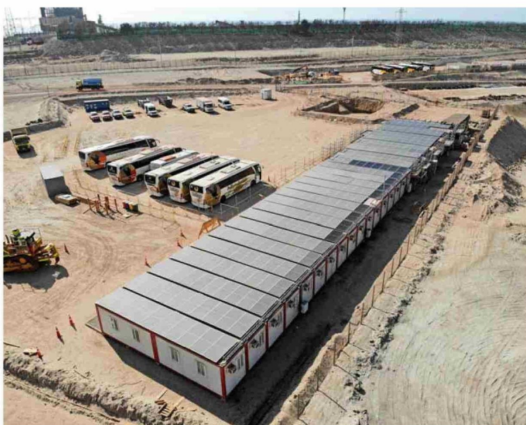
Unidades solares fotovoltaicas modulares, dispuestas en los techos de las instalaciones de faena, sustituyen a los generadores de electricidad a diésel.
