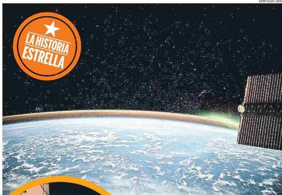
LA IONÓSFERA ES UNA CAPA ATMOSFÉRICA CARGADA DE ELECTRONES.
